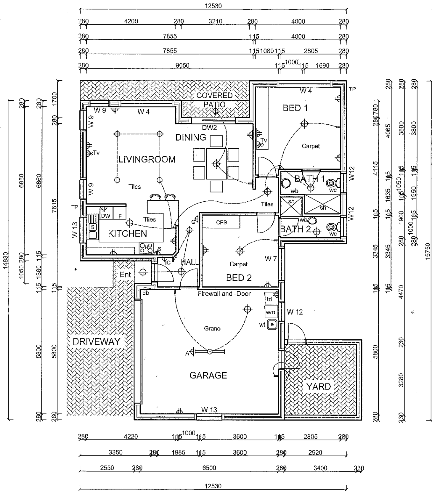
TYPE UD - FLOORPLAN - 1:100
